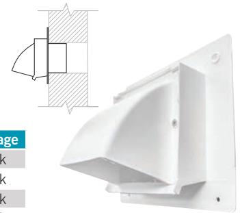
WC401
